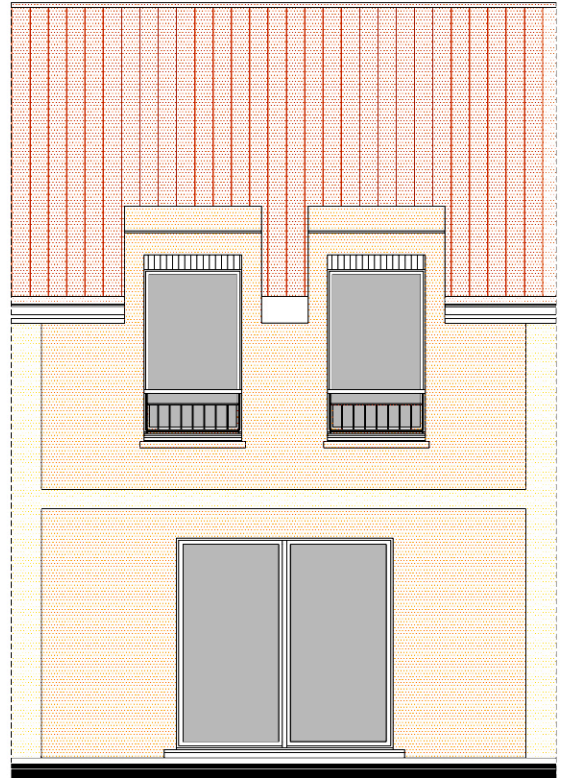
Façade JARDIN
